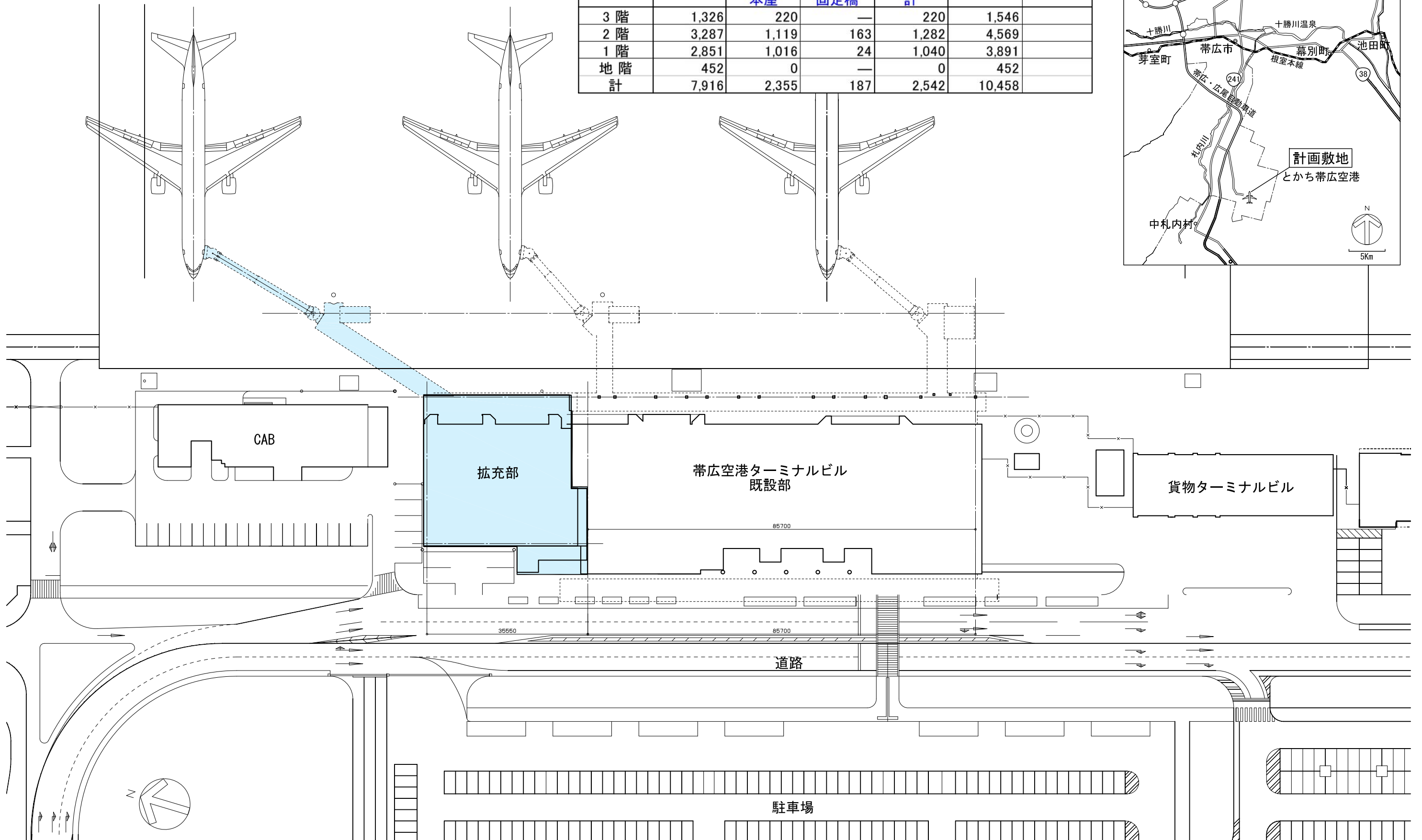
敷地案内図・配置図
